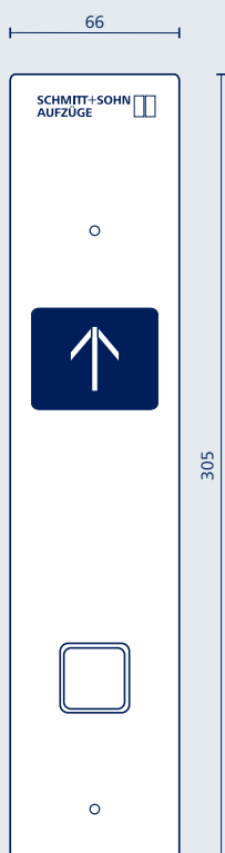
BT 1 Bedientableau mit einem Ruftaster und Weiterfahrtpfeilen
