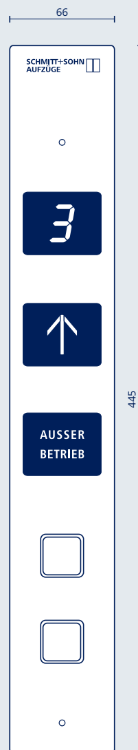
BT 4 Bedientableau mit zwei Ruftastern, Weiterfahrts- pfeilen und 2 LED- Anzeigen für Sonder- funktionen
