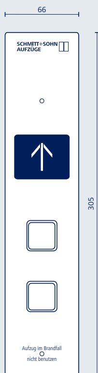
BT 2 Bedientableau mit zwei Ruftastern, Weiterfahrtpfeilen und Beschriftung
